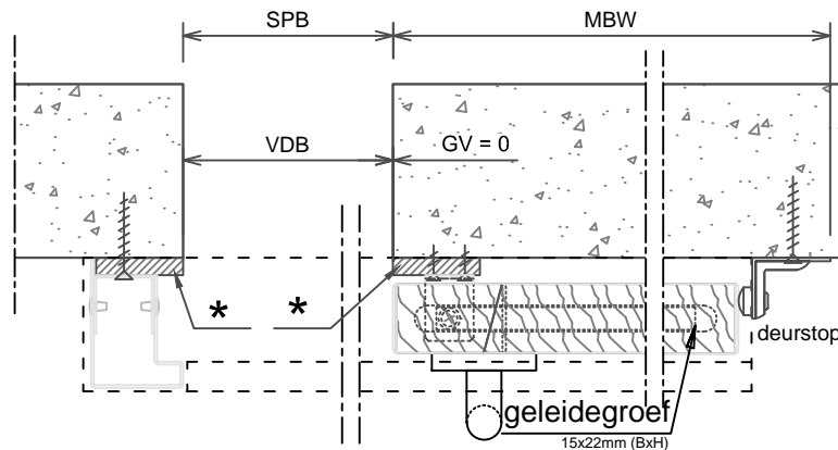
Horizontale Doorsnede GV=0
