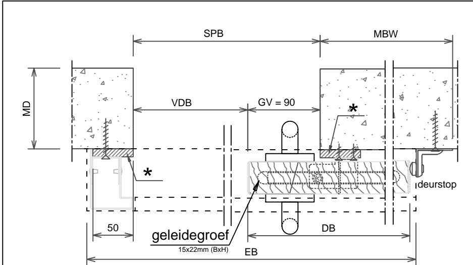
Horizontale doorsnede GV=90
